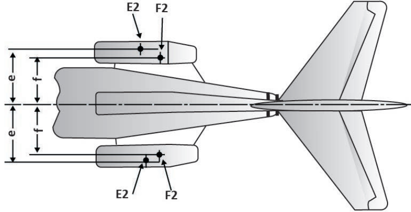
Görsel 5.38: Motorların simetri kontrolü
