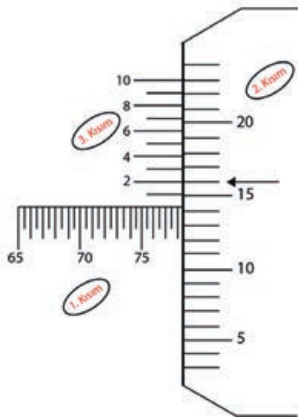
Görsel 2.70: 1/1000 mm'lik mikrometre okuması
