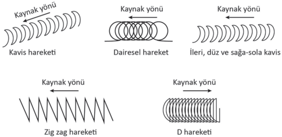
Görsel 4.22: Kaynak dikiş hareketleri örneği
