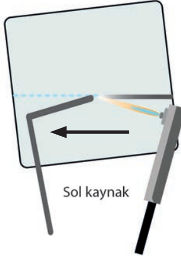
Görsel 4.23: Sol kaynak uygulaması
