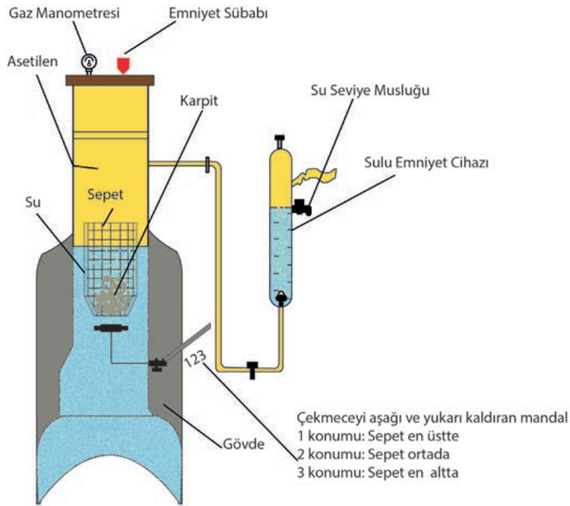
Görsel 4.17: Asetilen kazanı ve sulu güvenlik
