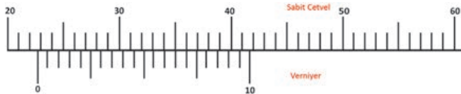
Görsel 2.47: 1/20 mm'lik kumpasta ölçü okuma
