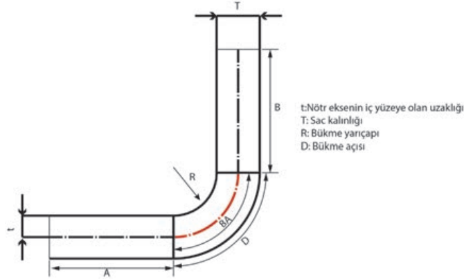
Görsel 2.105: Bükme hesabı
