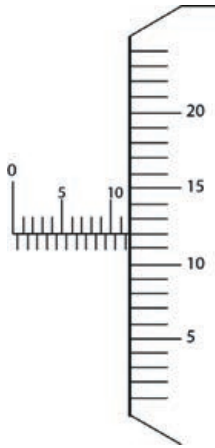
Görsel 2.72: 1/100 mm'lik mikrometre okuması
