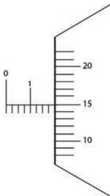
Görsel 2.79: 1/1000 inch'lik mikrometre okuması
