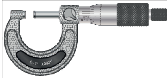
Görsel 2.62: 1/10000" mikrometre
