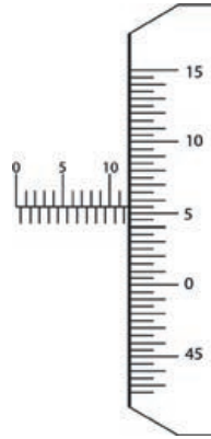
Görsel 2.76: 1/200 mm'lik mikrometre okuması
