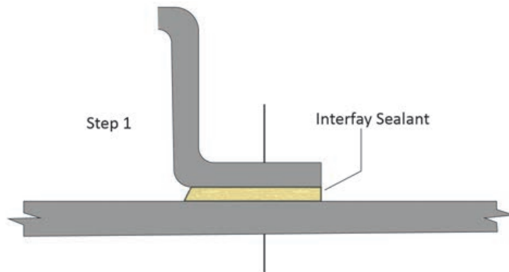
Görsel 6.5: Basıncı sıvı contalama işlemi
