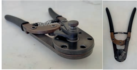
Görsel 3.19: Perçin kesme makası
