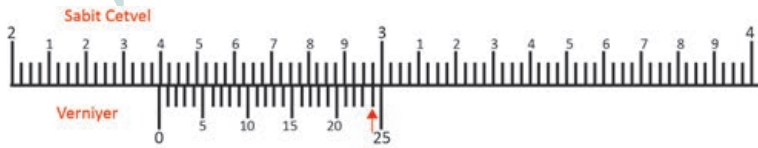
Görsel 2.58: 1/1000 inch'lik kumpasta ölçü okuma
