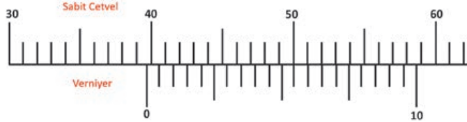
Görsel 2.46: 1/20 mm'lik kumpasta ölçü okuma
