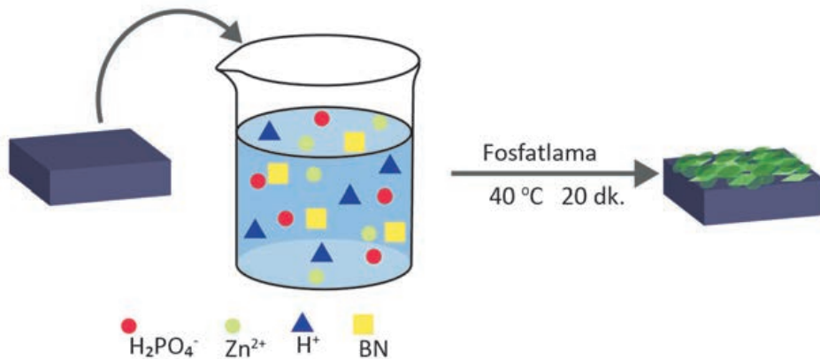
Görsel 5.22: Fosfat kaplama
