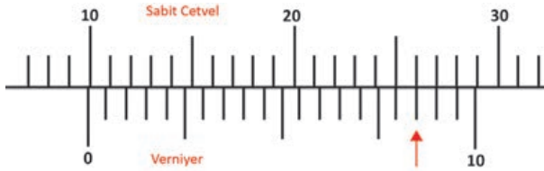
Görsel 2.38: 1/20 mm'lik kumpasta ölçü okuma
