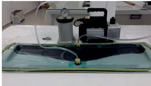
Görsel 1.17: Reçine transfer kalıplama yöntemi
