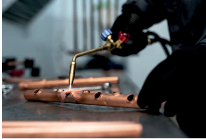
Görsel 4.7: Üfleç
