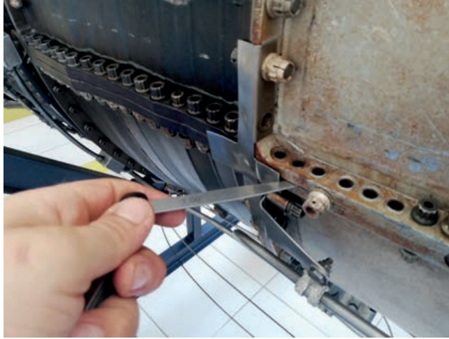
Görsel 2.109: Sentil uygulaması
