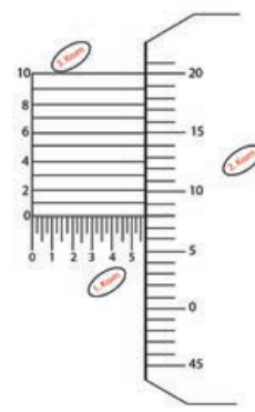
Görsel 2.69: 1/10000 inch'lik mikrometre
