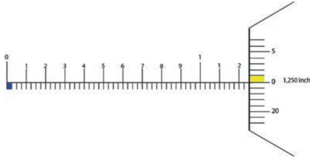
Görsel 2.64: Inch(Inch) mikrometre
