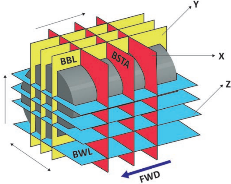
Görsel 5.8: Uçağın referans düzlemleri
