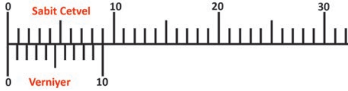
Görsel 2.33: Mm'lik kumpas
