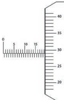
Görsel 2.76: 1/100 mm'lik mikrometre okuması
