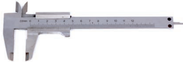
Görsel 2.29: Kumpas
