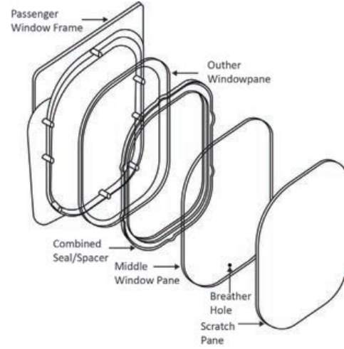
Görsel 5.65: Yolcu pencereleesi detay resmi
