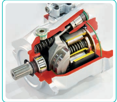
Görsel 2.9: Pistonlu pompanın iç yapısı
