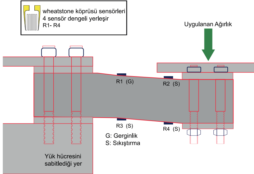
Şekil 6.2: Wheatstone köprüsü ve dört sensörün bileşimi
