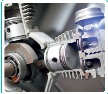
Görsel 2.15: Pistonlu kompresörün iç yapısı
