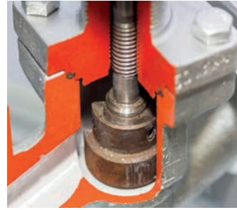
Görsel 1.8: Glob vana
