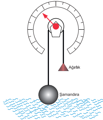
Şekil 3.10: Şamandıralı seviye ölçer
