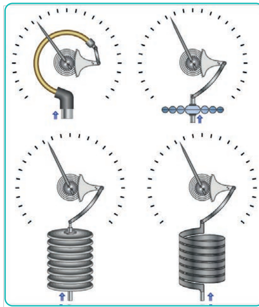
Görsel 3.3: Bourdon manometre iç dizaynı
