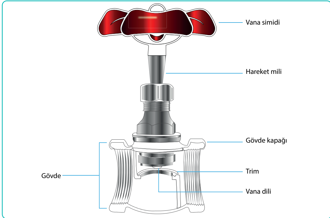
Şekil 1.1: Glob vana aparatları
