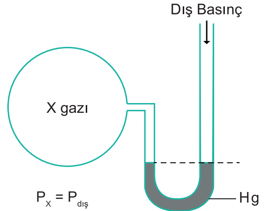
Şekil 3.3: Açık uçlu manometre
