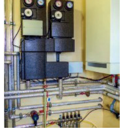
Görsel 4.9: Isıtma sisteminin çevre donanımı
