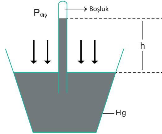
Şekil 3.6: Barometre
