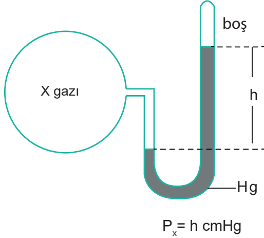
Şekil 3.1: Kapalı uçlu manometre
