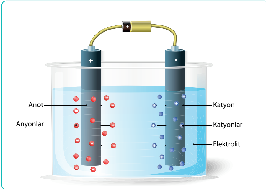
Görsel 9.7: Elektroliz düzeneği
