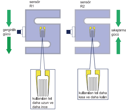
Şekil 6.1: Gerinim yük hücresi gövde yapısı
