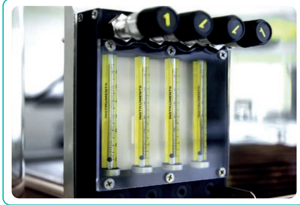
Görsel 3.10: Rotametre
