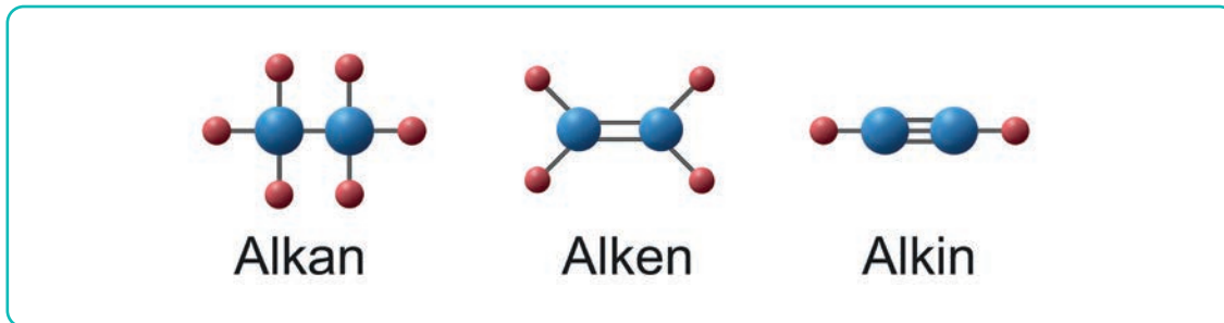
Görsel 10.3: Alkan, alken ve alkin molekül yapısı
