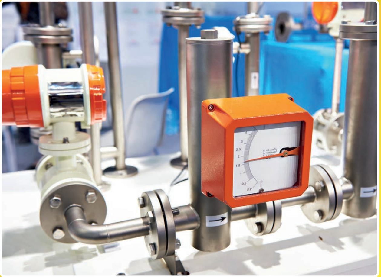
Görsel 3.8: Debimetre
