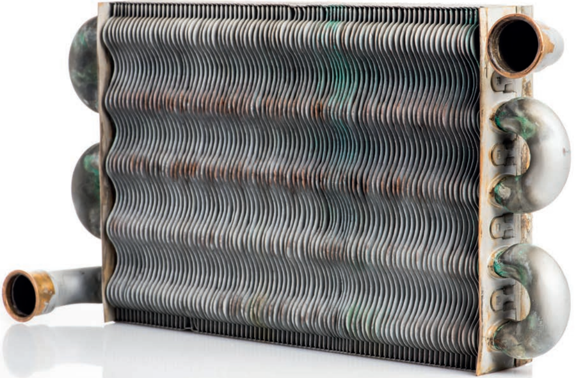
Görsel 4.7: Serpantinli ısı değıştirci
