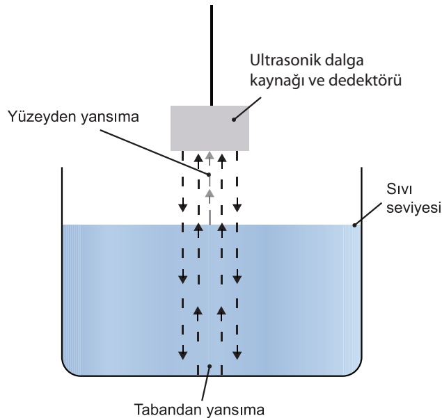
Şekil 3.11: Ultrasonik seviye ölçer
