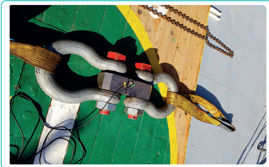
Görsel 6.3: Yük testi için iki kelepçeli ve ağ askılı yük hücresi
