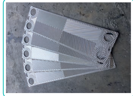
Görsel 4.6: Isı değıştirci levhalar
