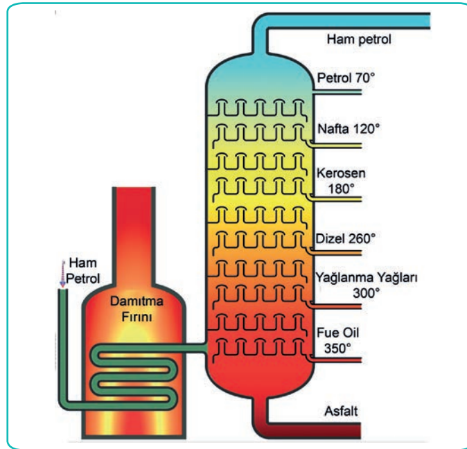
Görsel 10.4: Petrol damıtma kulesi
