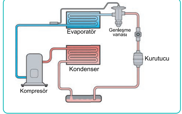
Görsel 5.6: Çiller soğutma sistemi temel elemanları
