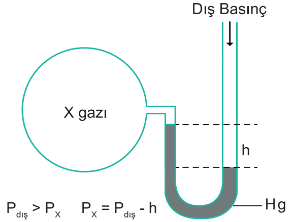
Şekil 3.5: Açık uçlu manometre
