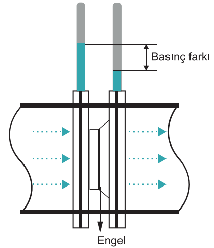
Şekil 3.9: Fark Basınç Debimetre (orifis metre)
