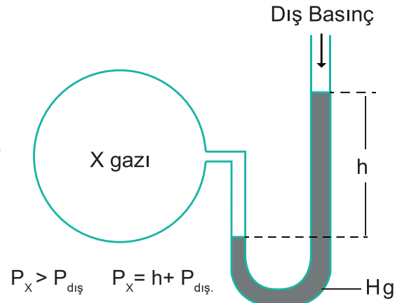
Şekil 3.4: Açık uçlu manometre
