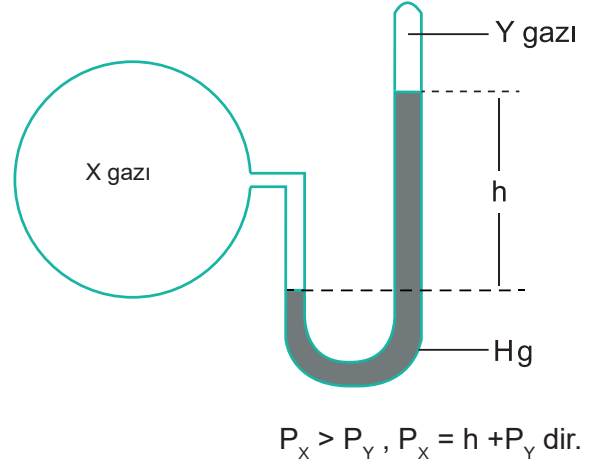
Şekil 3.2: Gaz bulunan kapalı uçlu manometre
