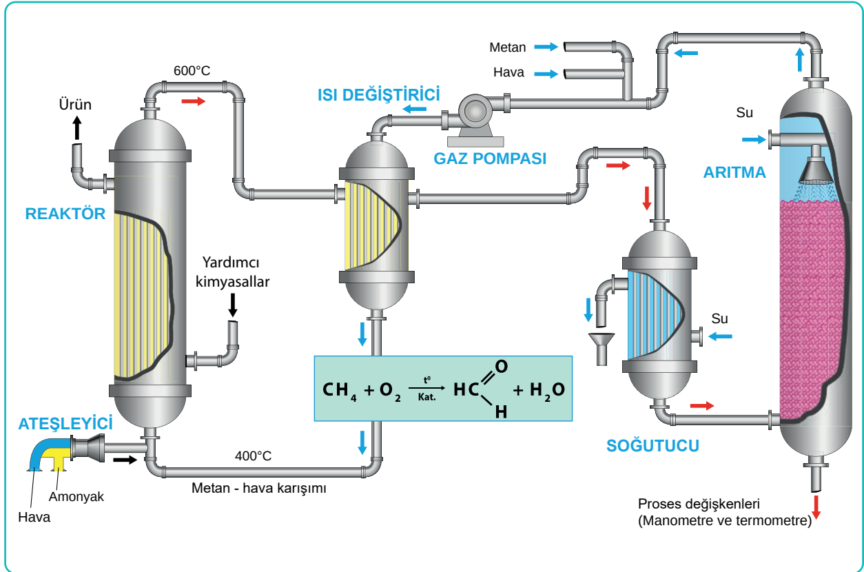
Görsel 7.4: Formaldehit prosesinde bulunan reaktör ve çevre donanımı
