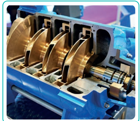
Görsel 2.10: Santrifüj pompanın içinden kesit
