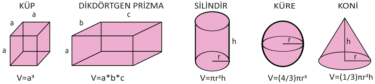
Şekil 2.1: Hacim formülleri
