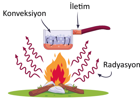
Görsel 3.9: Kondüksiyon
