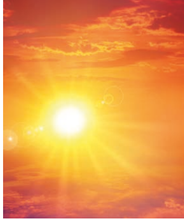
Görsel 3.14: Işıma
