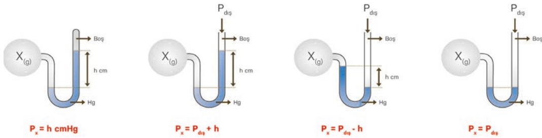
Şekil 2.2: Kapalı ve açık uçlu manometrelerde P_{x(gaz)} miktarının ölçüm formülleri
