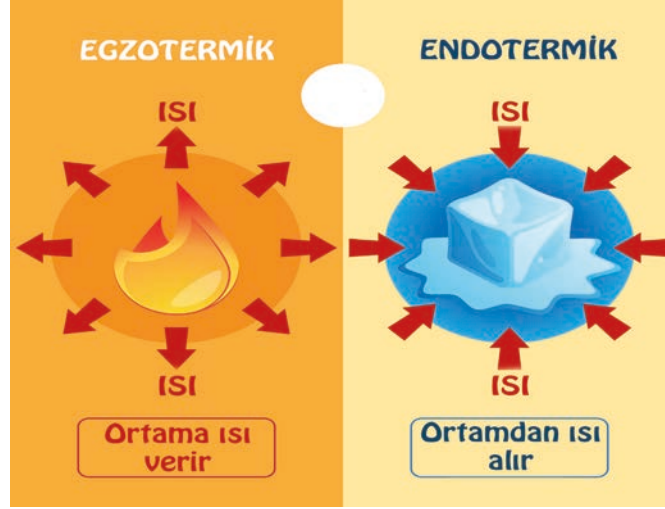
Görsel 3.4: Reaksiyon
