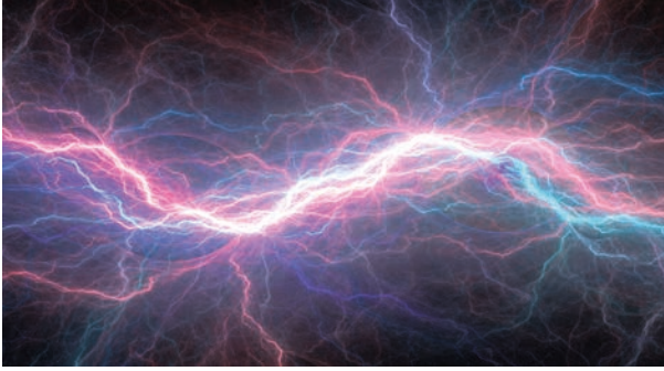
Görsel 1.1: Elektrik
