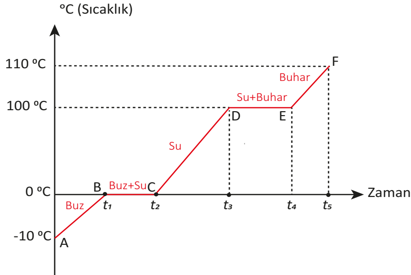
Grafik 2.1: Katı buzun sıcaklığı
