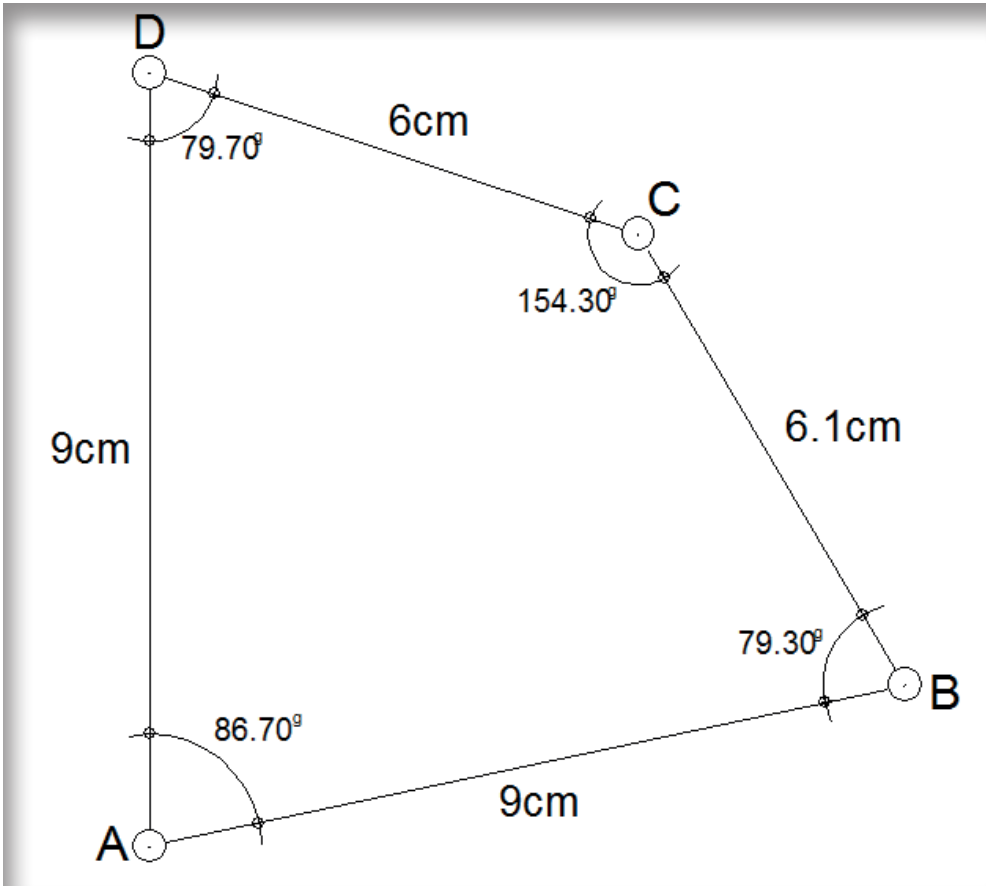
Görsel 1.6. Minkale ile dörtgen çizimi
