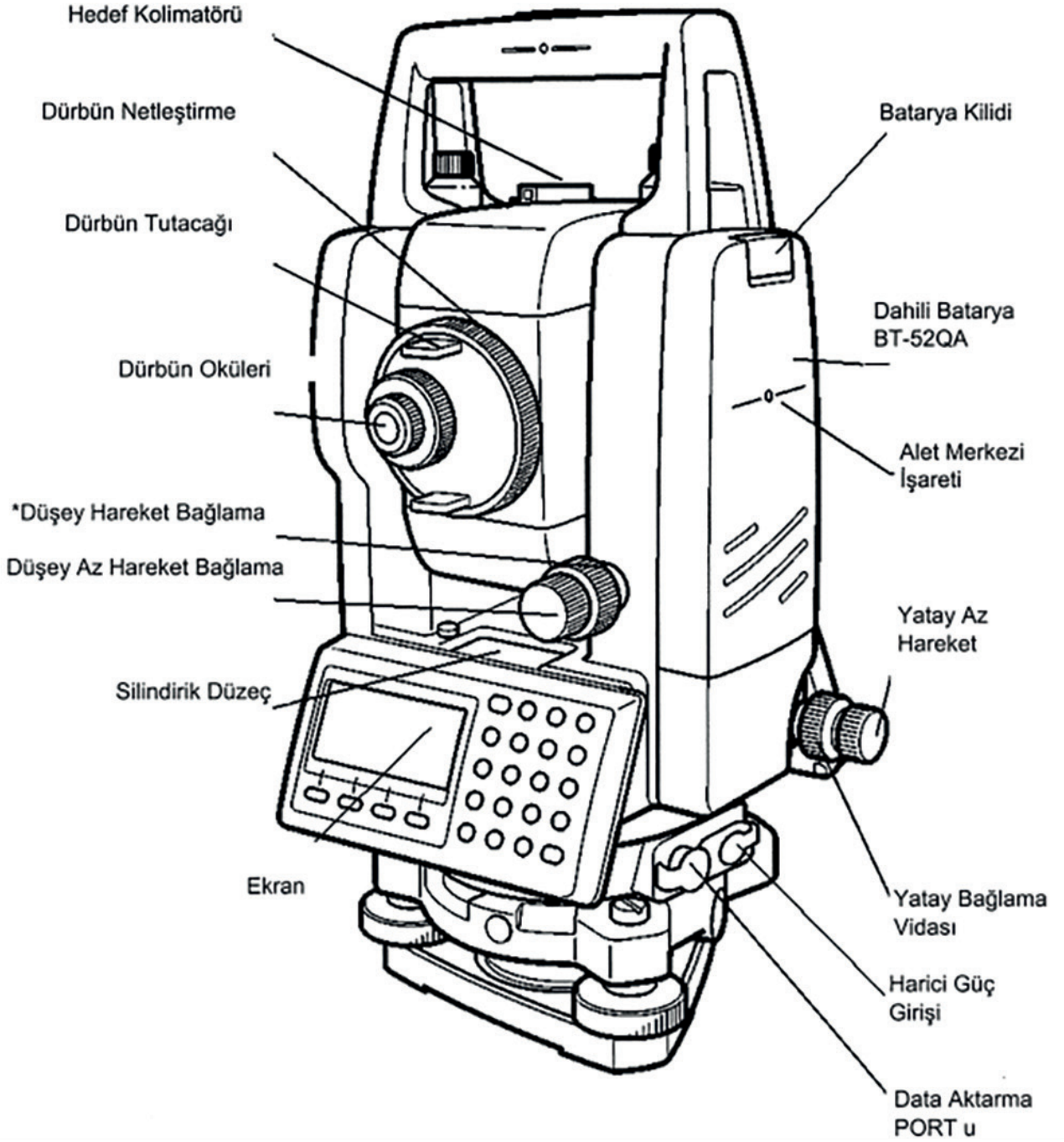
Görsel 3.2: Elektronik alet parçaları
