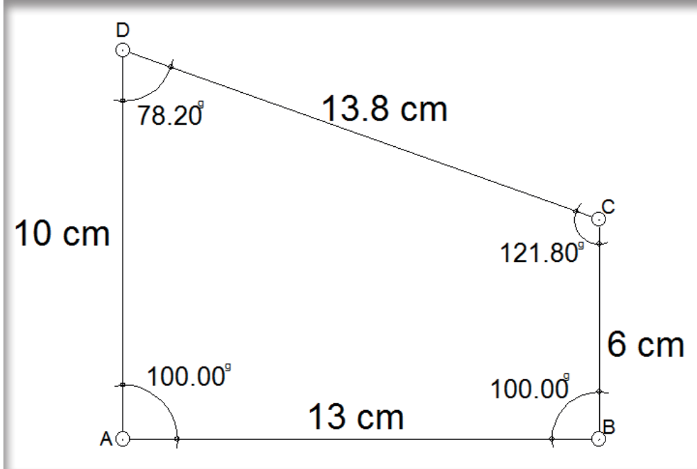
Görsel 1.5: Minkale ile Yamuk Çizimi
