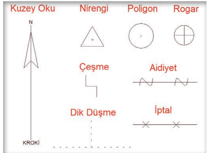
Görsel 1.1: Krokilerde kullanılan işaretler
