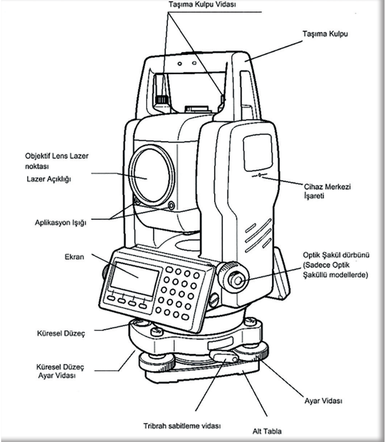
Görsel 3.1: Elektronik alet parçaları
