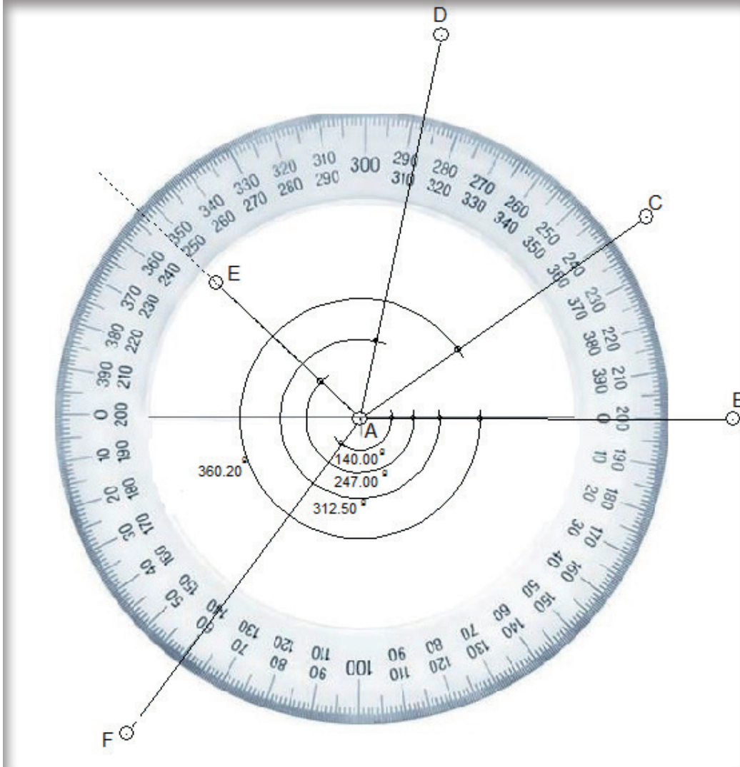
Görsel 1.3: Minkale ile Açı ölçme
