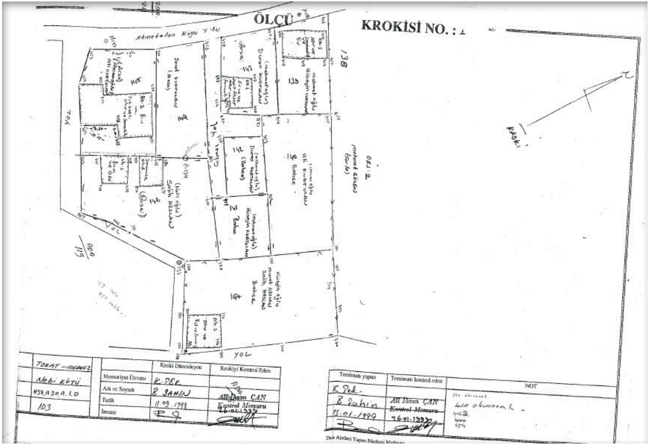
Görsel 1.2: Ölçü krokisi
