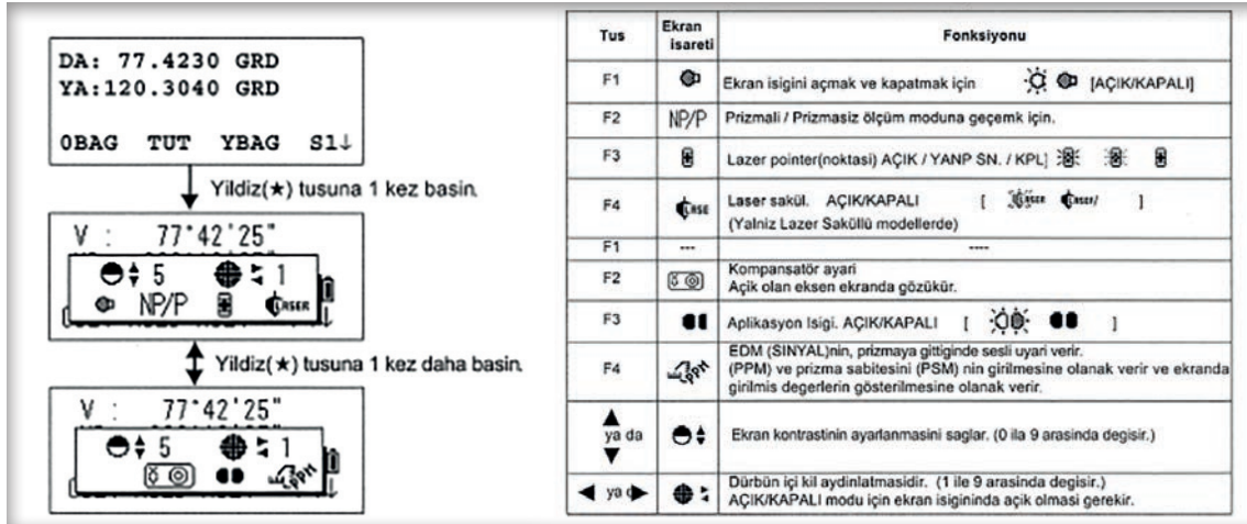
Görsel 3.5: Ekran tuşları ve fonksiyonları
