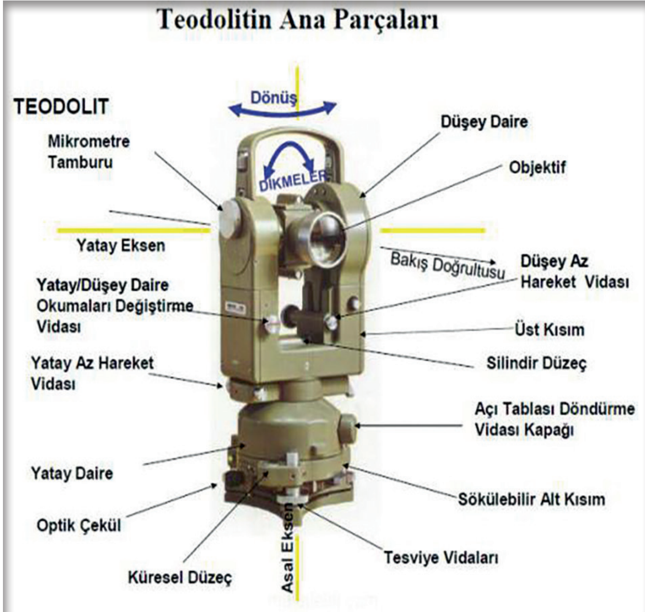
Görsel 2.8: Teodolit ana parçaları
