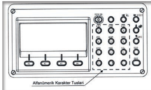
Görsel 3.4: Çalıştırma Tuşları
