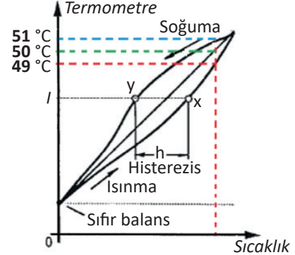
Grafik 1.5: Histerezis grafiği
