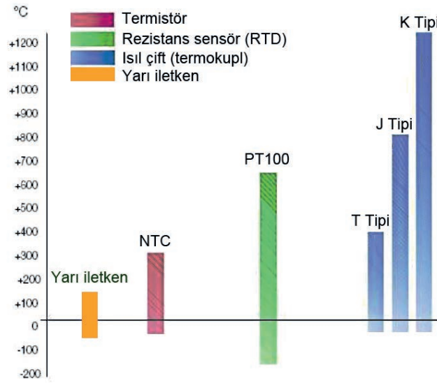
Grafik 1.6. Sıcaklık ölçümünde sensör seçimi
