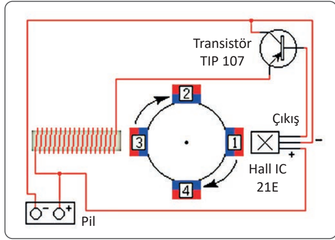
Şekil 1.56: Devre şeması
