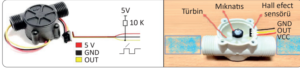
Şekil 2.6: YF-S201 su akış sensörünün bağlantı şeması
