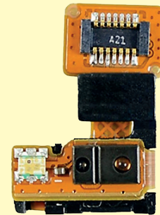
Fotoğraf 2.1 Yakınlık sensörü
