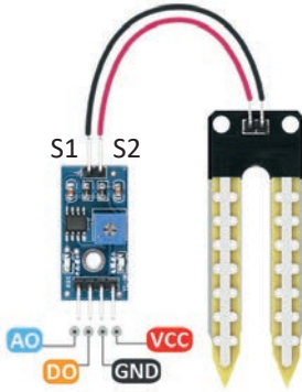
Şekil 2.29: Toprak sensörü ve bağlantı şeması
