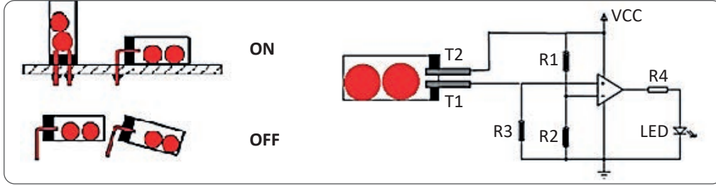
Şekil 2.8: SW520D eğim sensörü devresi
