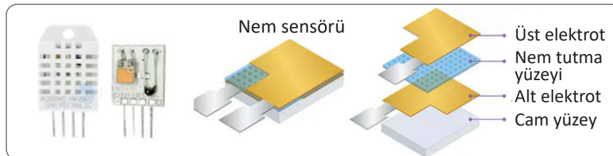
Şekil 2.19: DHT11'in iç yapısı
