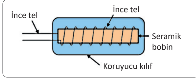
Şekil 1.46: Elektrik direnç termometresinin yapısı
