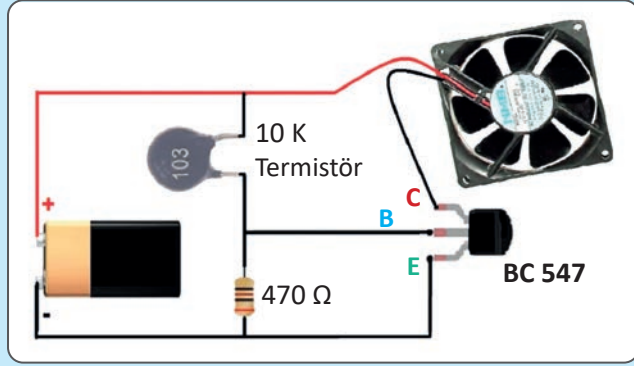
Şekil 1.44: Devre şeması
