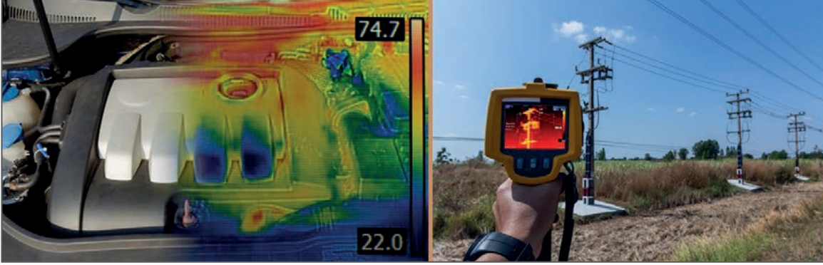
Fotoğraf 1.2: Kızılötesi termal görüntülemeyle motor ve enerji hatlarında önleyici bakım yapılması
