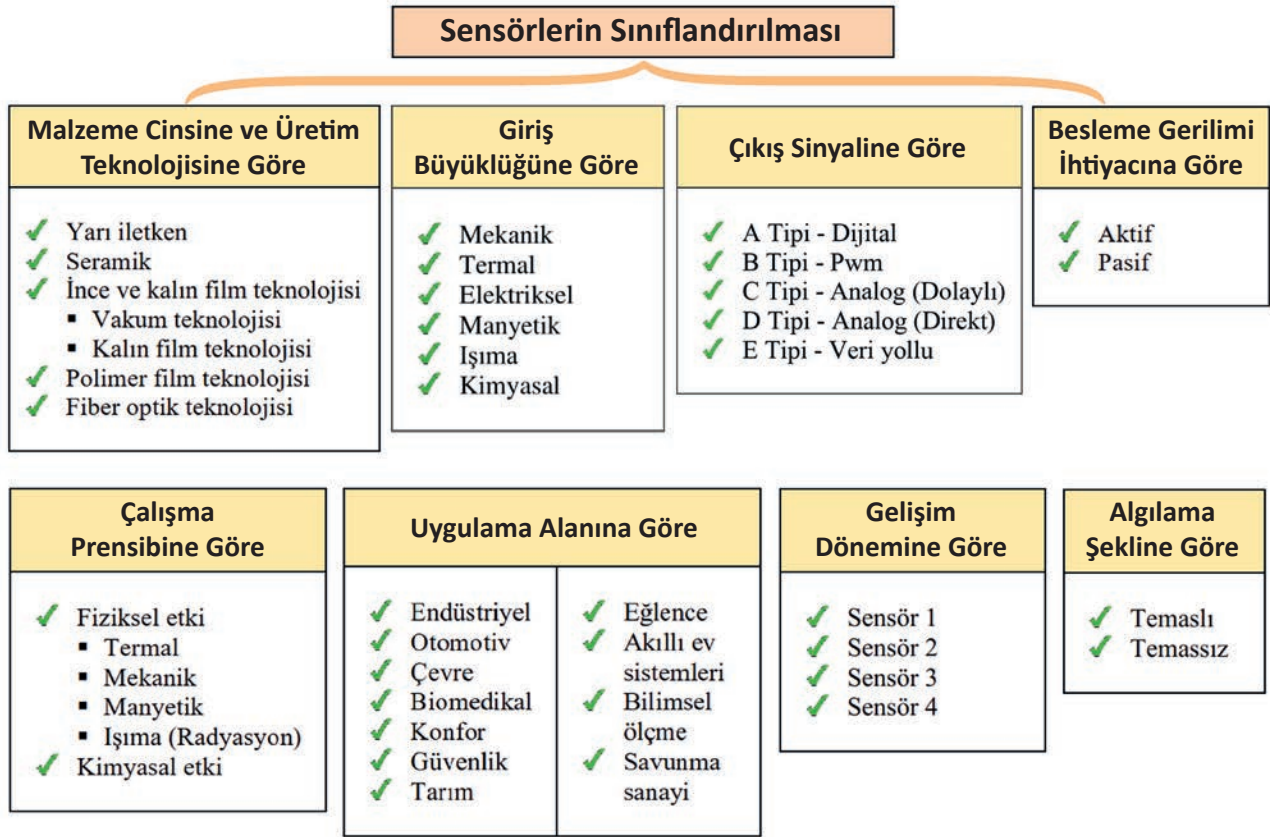
Şema 1.4: Sensörlerin özelliklerine göre sınıflandırılması
