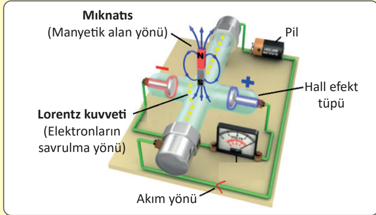
Şekil 1.53: Lorentz kuvveti
