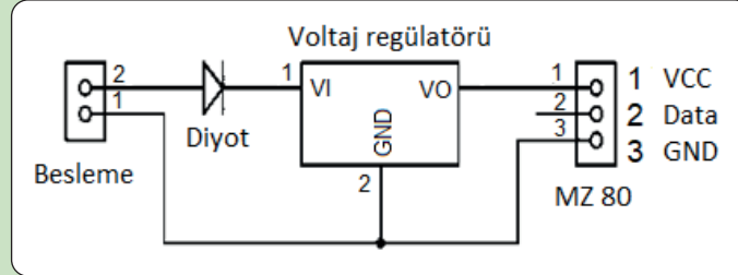
Şekil 2.43: Kızılötesi (IR) cisim algılama sensörünün beslenmesi
