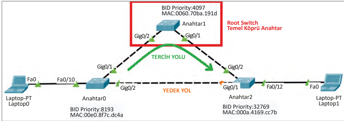
Görsel 8.25: BID öncelik değeri en küçük olan anahtar temel köprü anahtardır.
