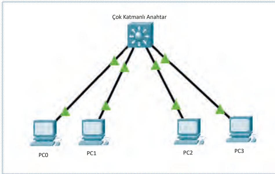
Görsel 9.1: Üçüncü katman anahtarlama cihazı bağlantısı
