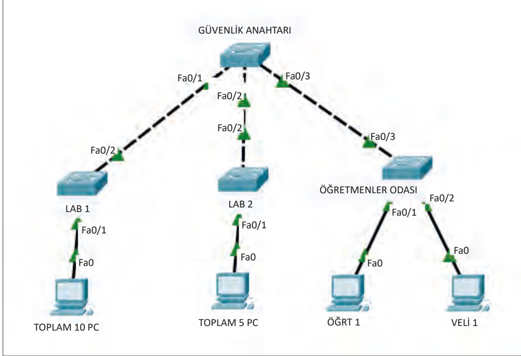
Görsel 10.20: Anahtar güvenliği topolojisi
