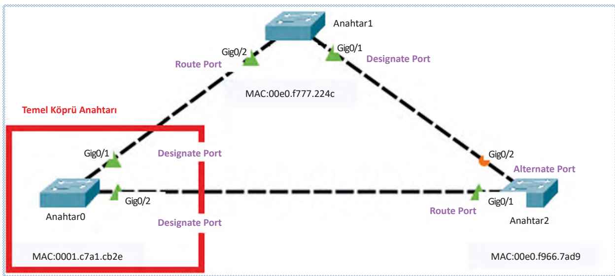
Görsel 8.39: STP arayüz rollerini
