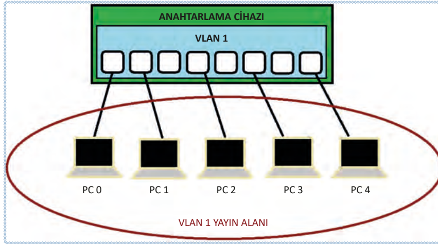
Görsel 7.1: VLAN 1 ile tek yayın alanı
