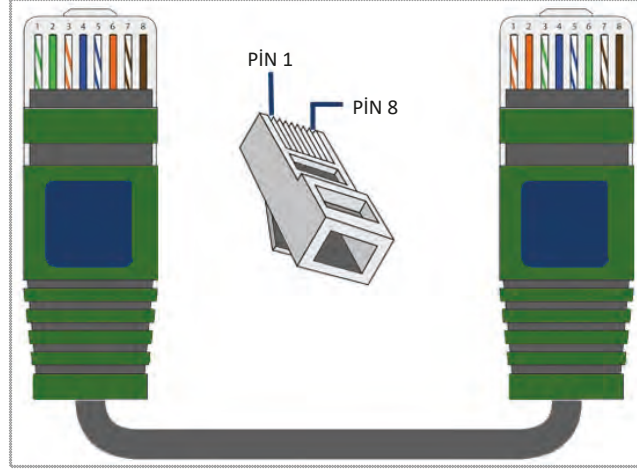
Görsel 2.7: Çapraz bağlantı türündeki ağ kablosu
