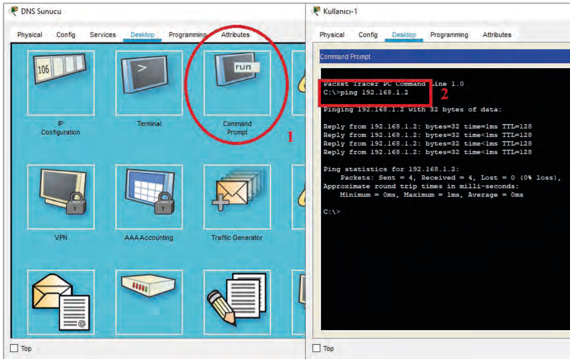
Görsel 3.13: Simülasyonun ping komutu ile test edilmesi
