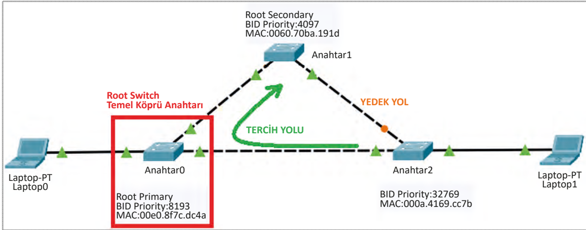
Görsel 8.28: Komutla bildirilen Anahtar, temel köprü anahtardır.
