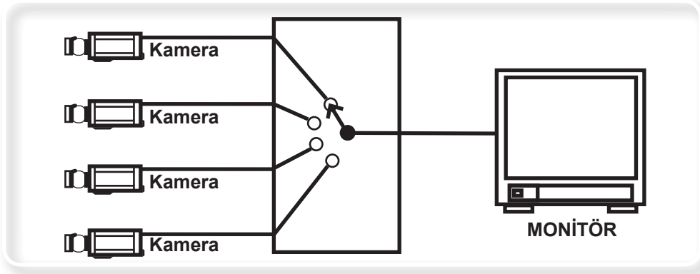
Şekil 1.2: Kapalı devre televizyon sistemi
